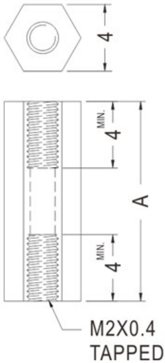
KHPL-26 结构图
