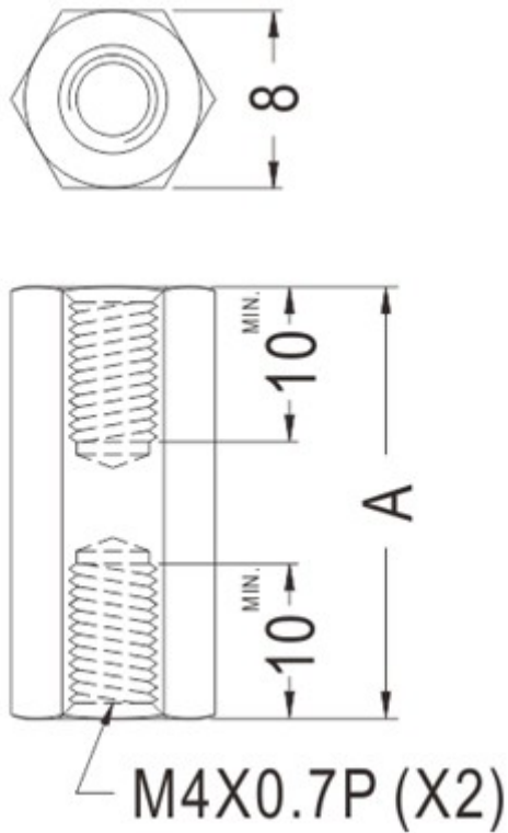
KHPL-29 结构图
