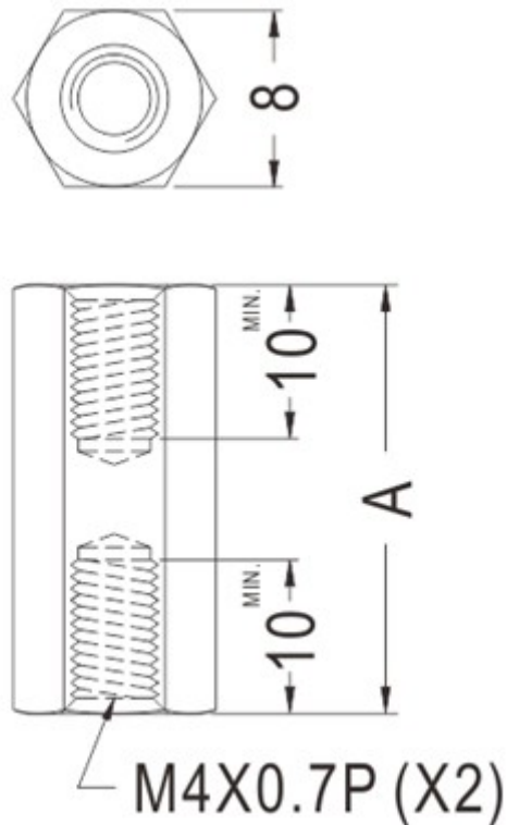
KHPL-28 结构图
