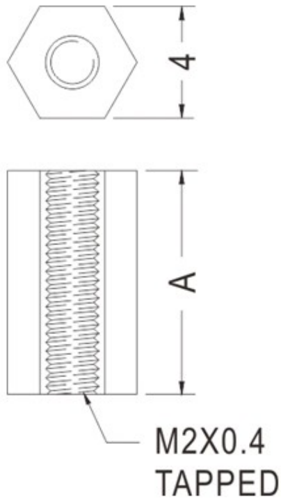
KHPL-07 结构图
