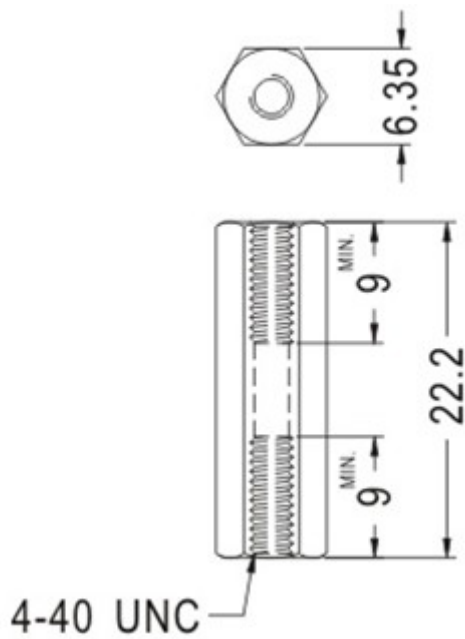
KHPL-01 结构图
