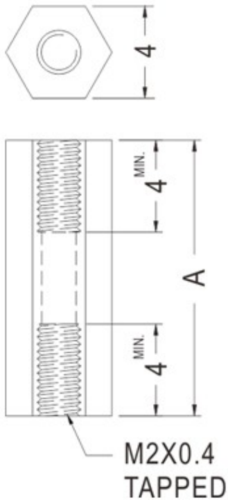
KHPL-23 结构图
