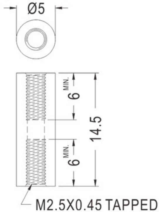
KHPL-03 结构图
