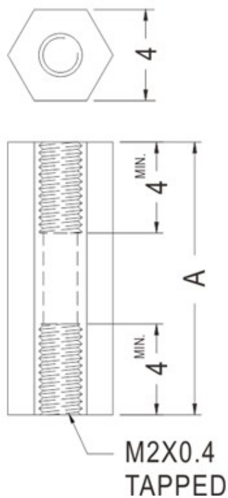
KHPL-13 结构图
