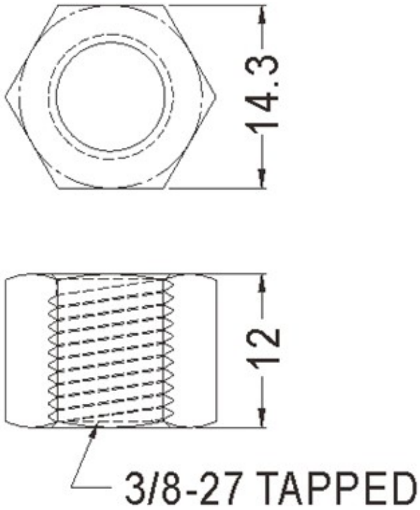
KHPL-27 结构图
