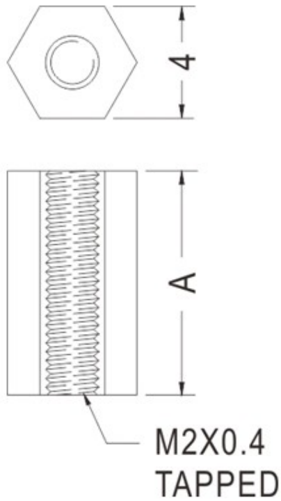
KHPL-06 结构图
