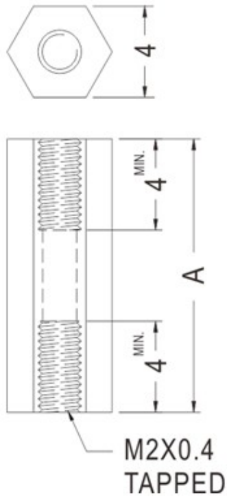
KHPL-19 结构图
