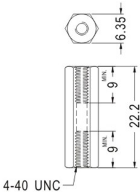
KHPL-02 结构图
