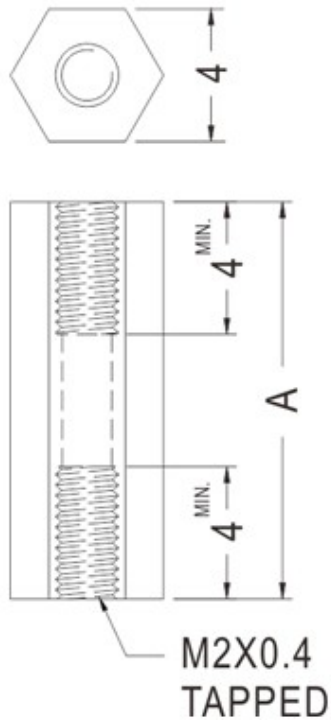
KHPL-10 结构图
