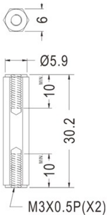
KHPL-30 结构图
