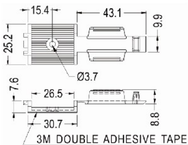
FCC-20 结构图
