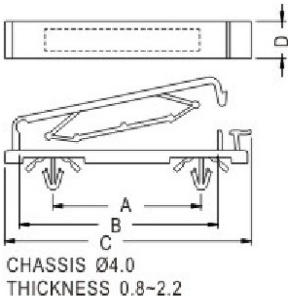
FCC-11 结构图
