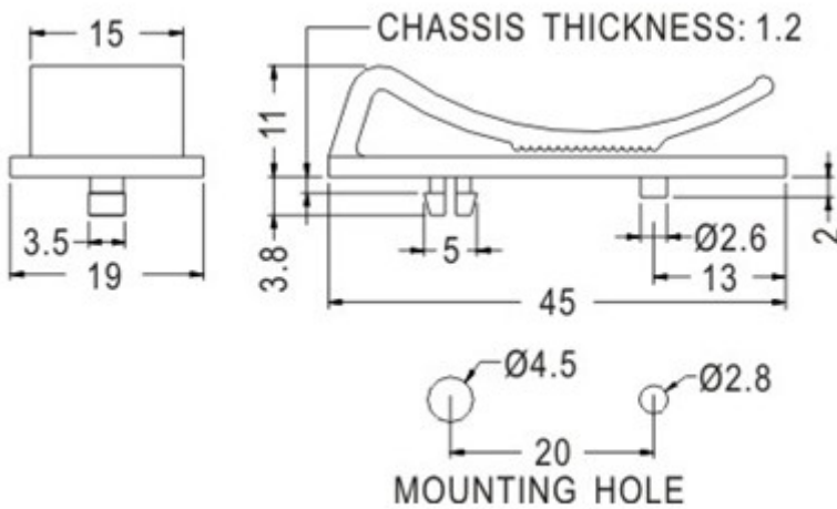
FCC-19 结构图
