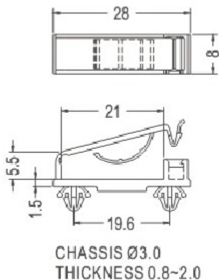
FCC-33 结构图
