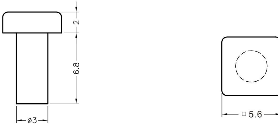
ACKS-1 结构图
